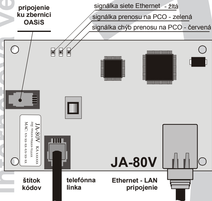
Obr. 1 Zapojenia komunikátora
