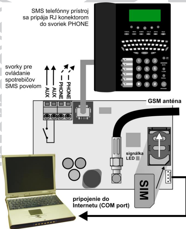
Obr. 1 Zapojenie komunikátora
